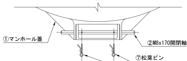
開閉軸 組立参考図
