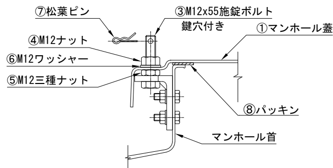
施錠ボルト組立参考図
