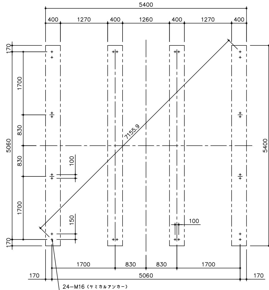
基礎伏図
