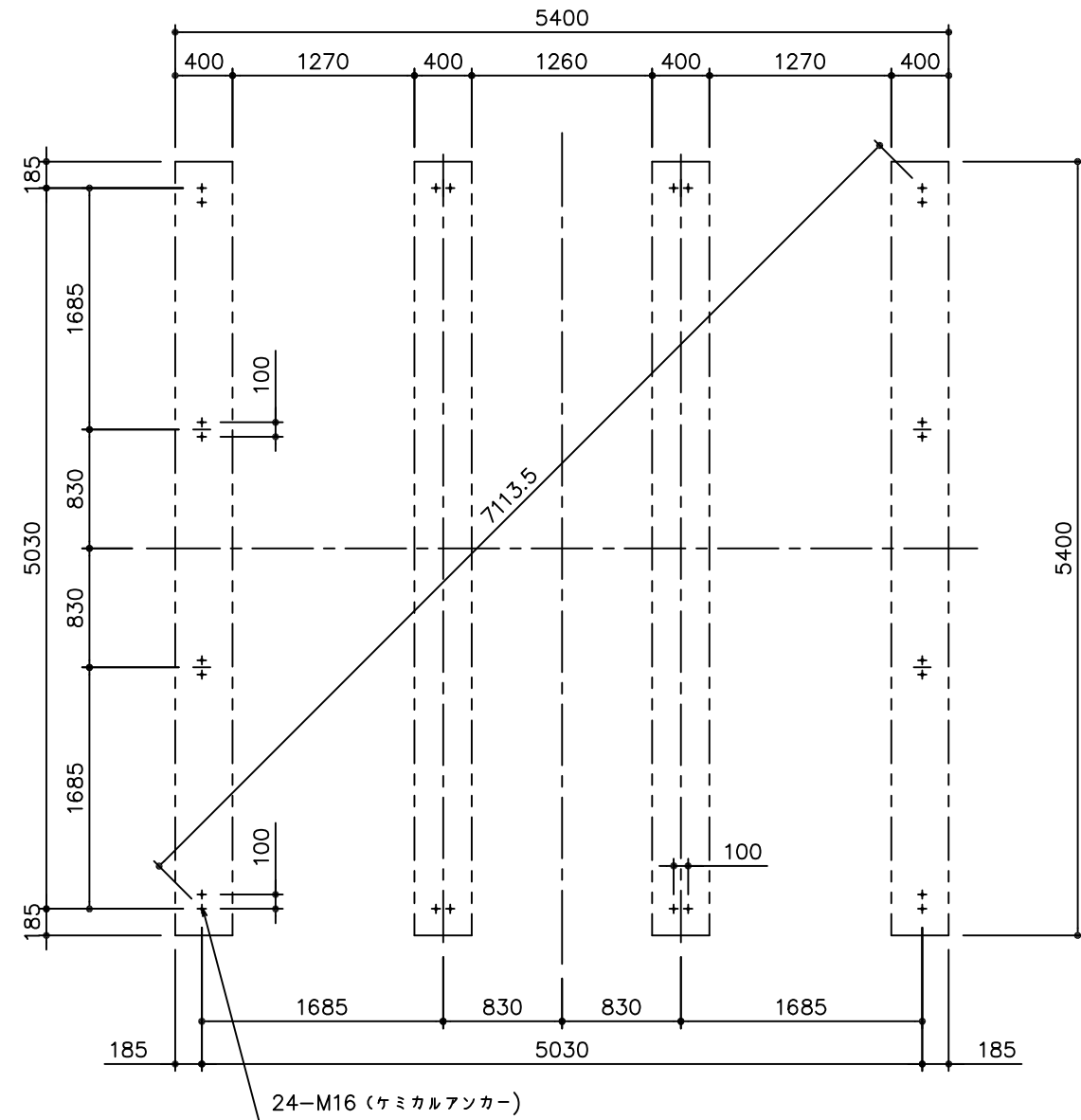
基礎伏図
