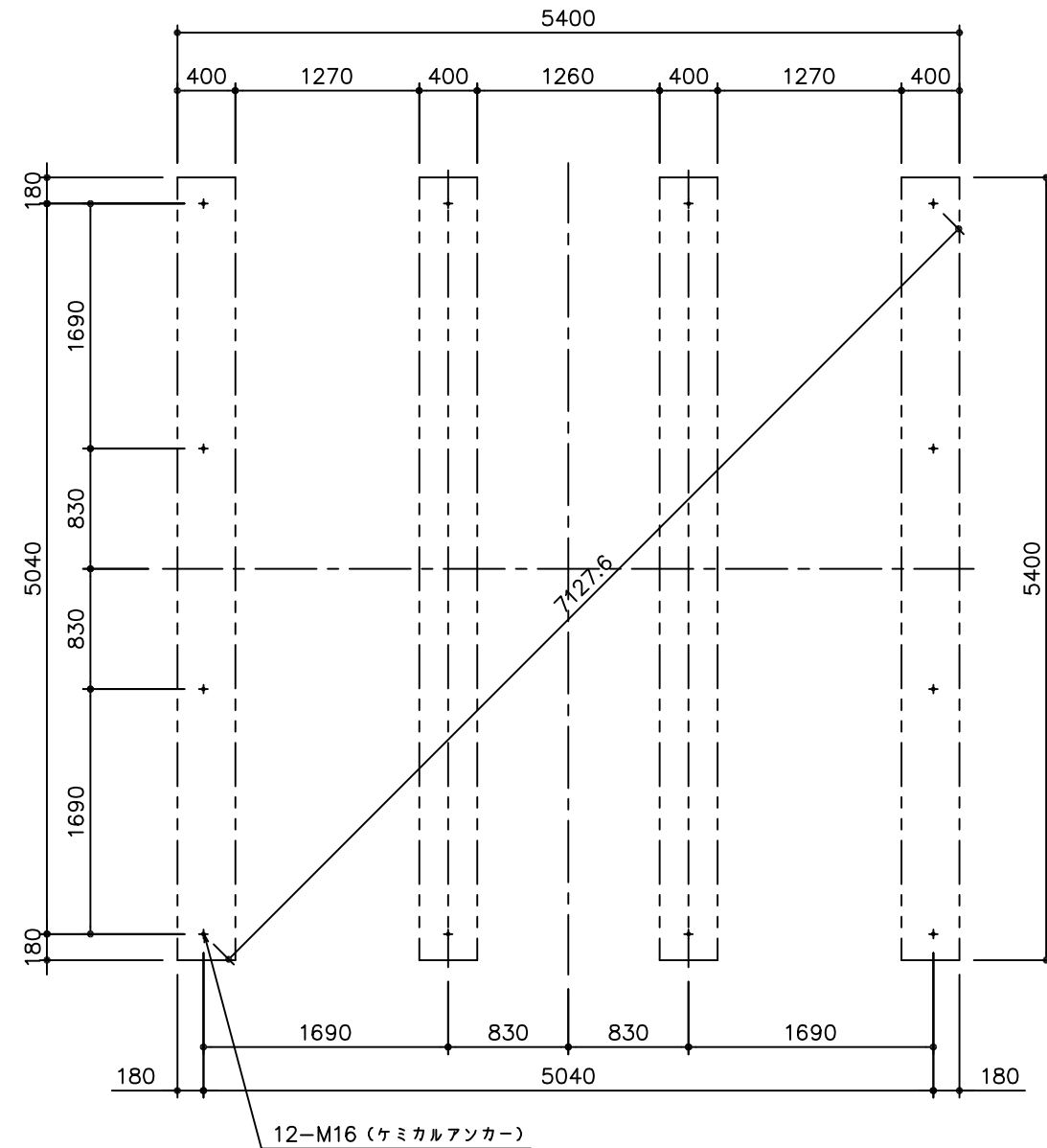
基礎伏図
