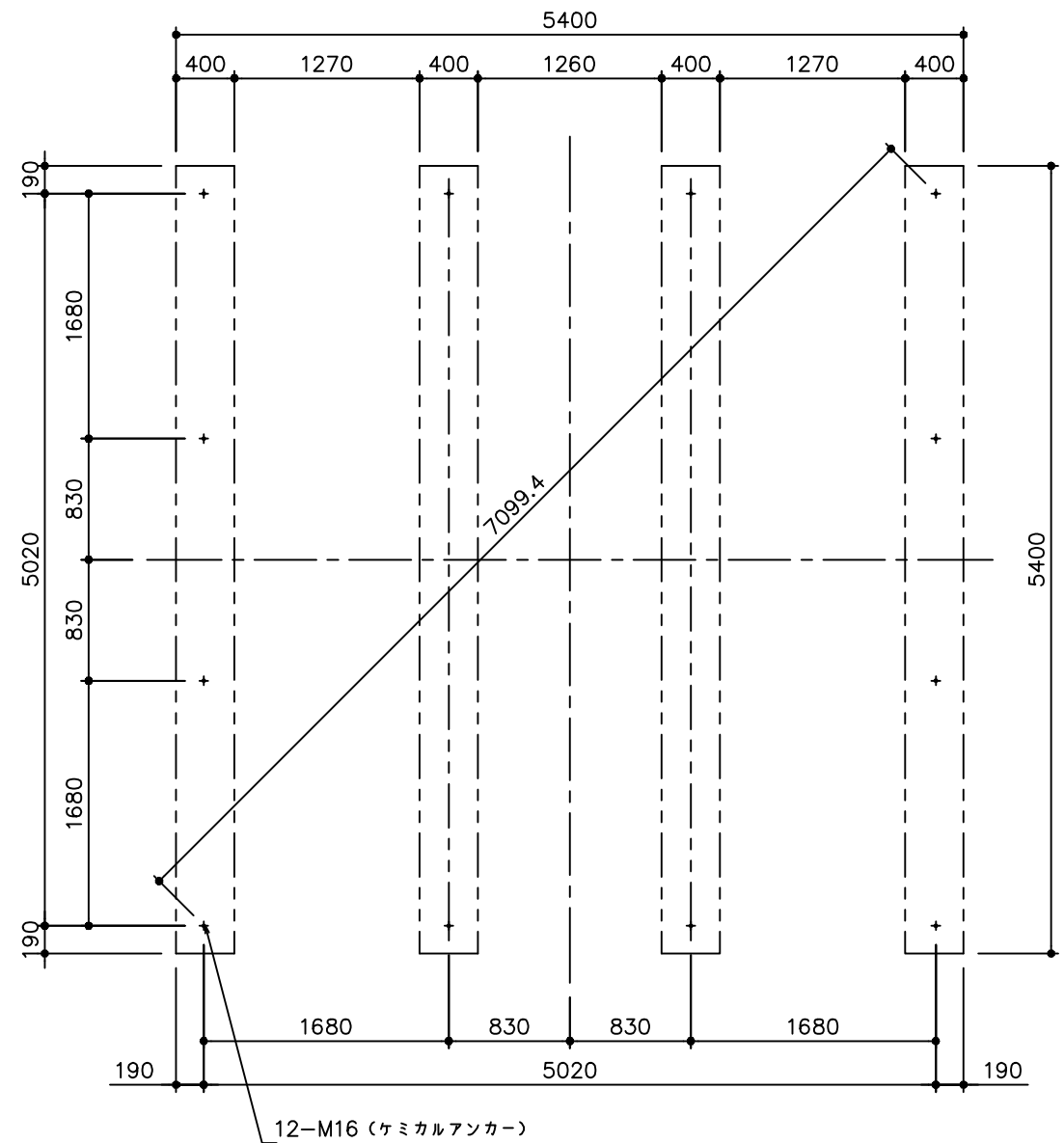
基礎伏図
