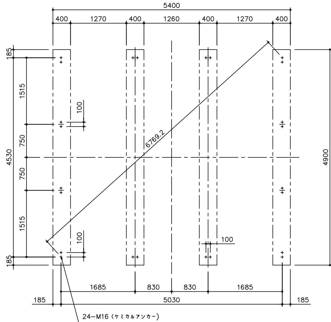
基礎伏図
