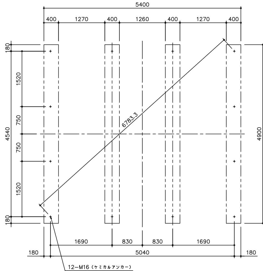
基礎伏図
