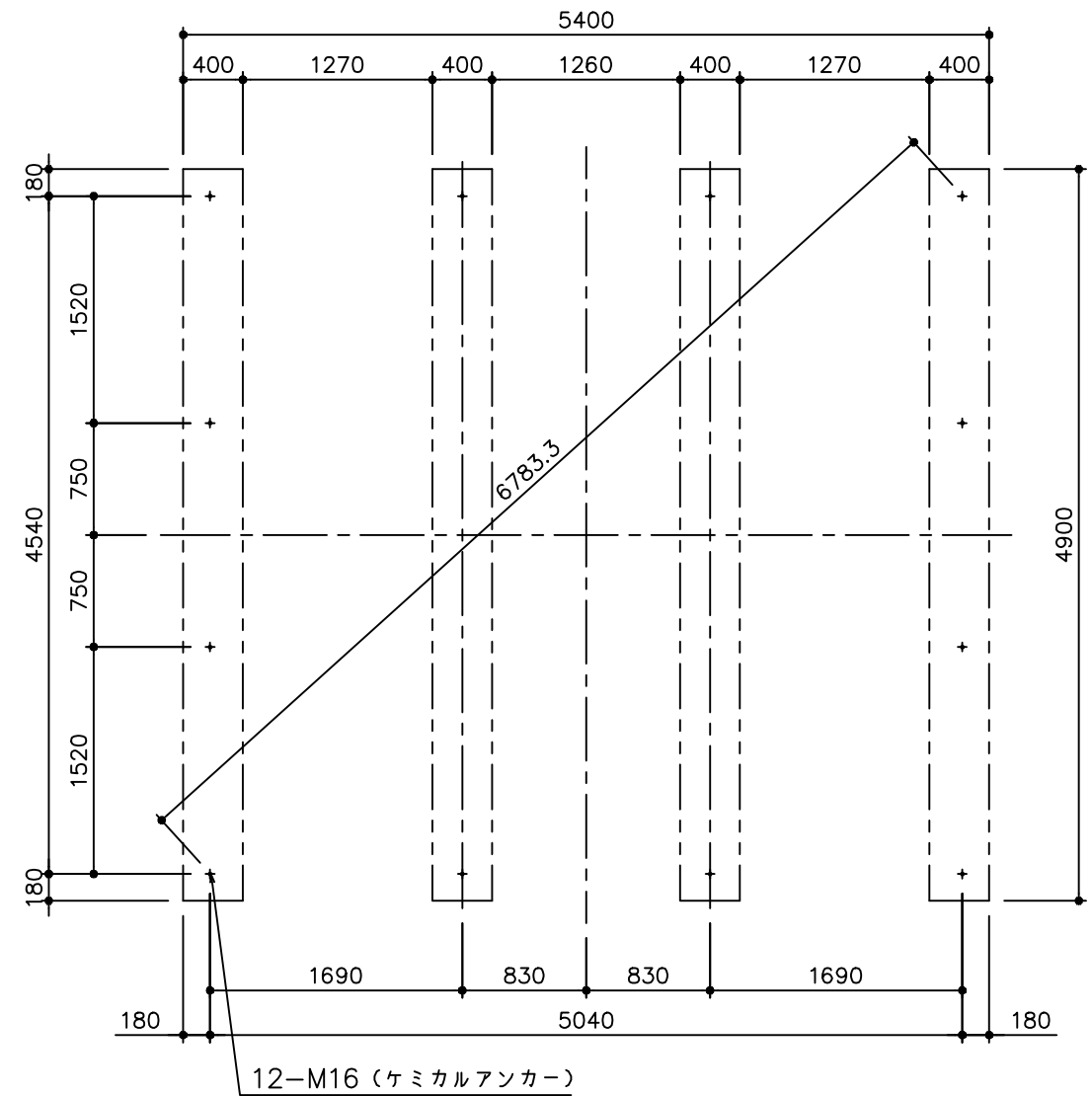
基礎伏図
