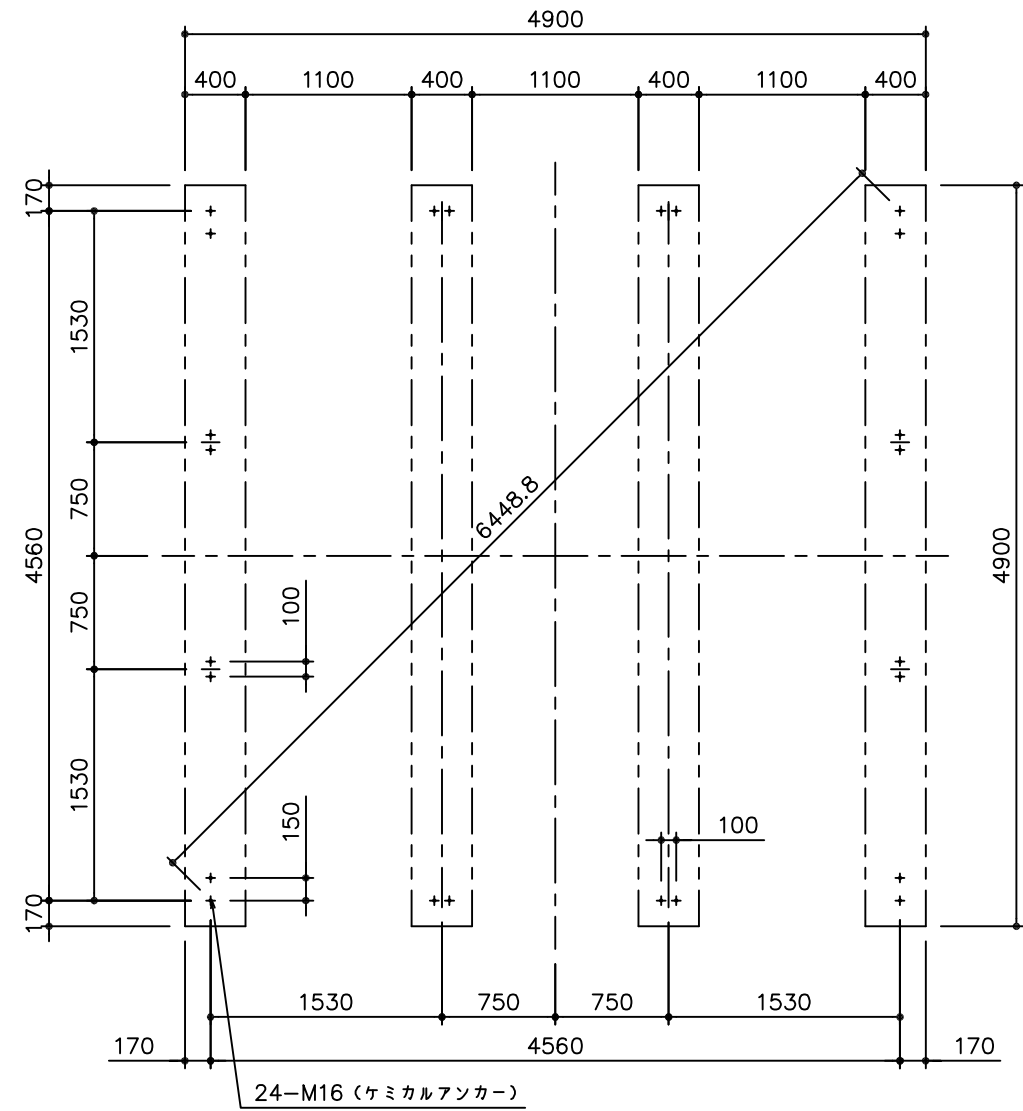
基礎伏図
