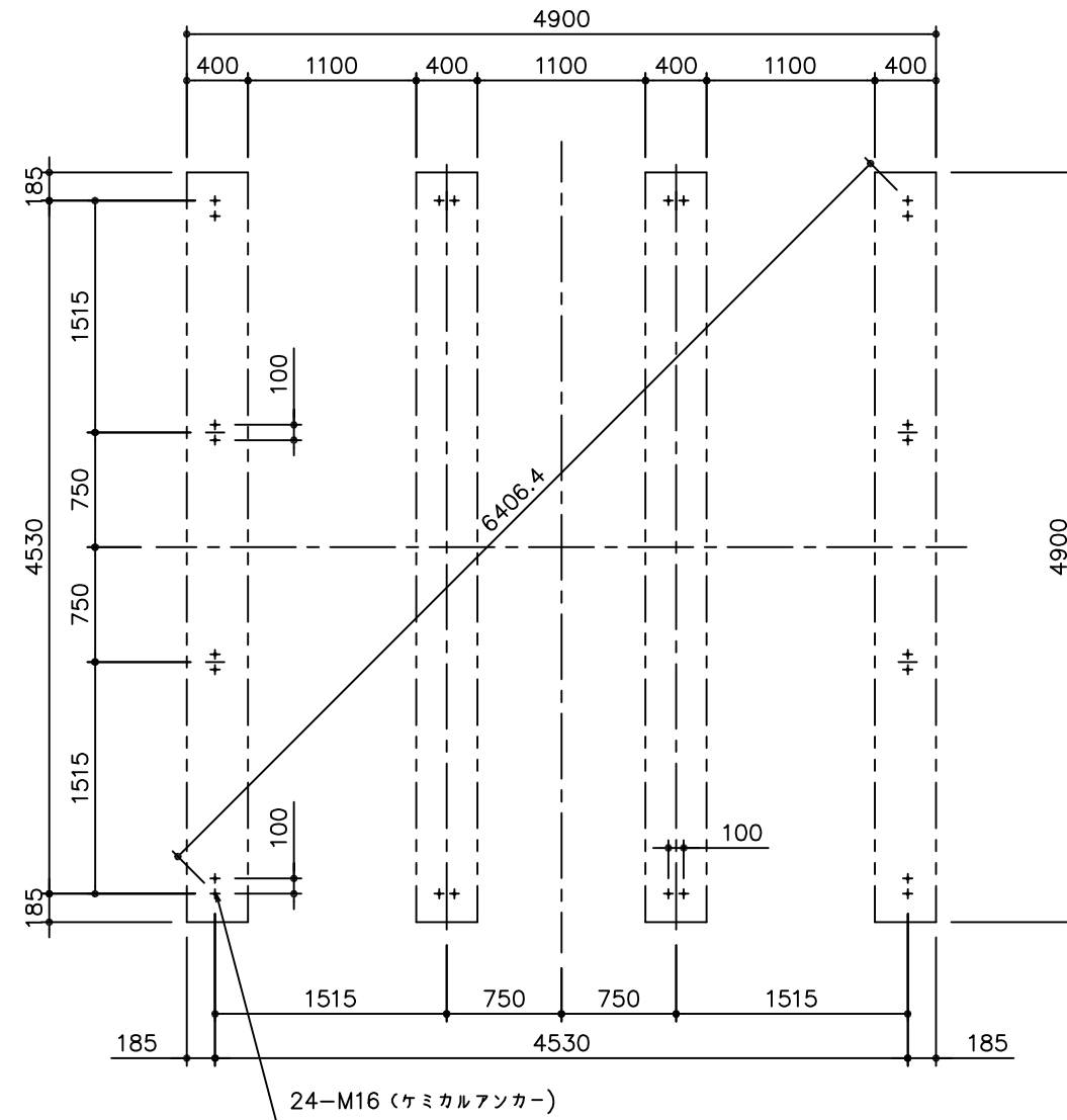
基礎伏図
