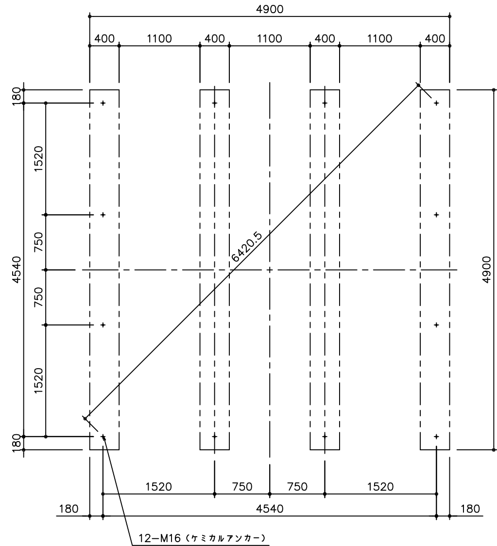
基礎伏図
