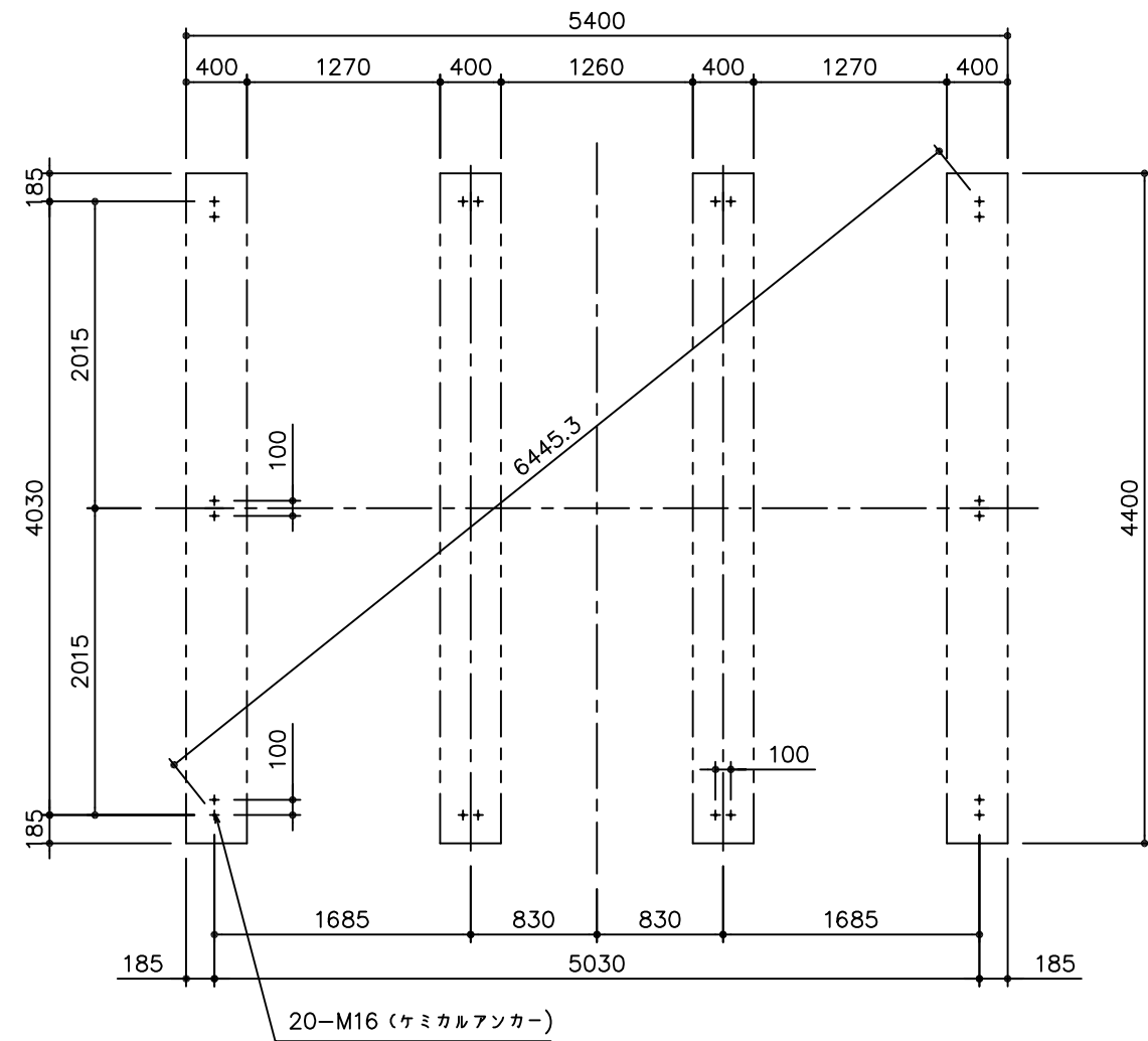
基礎伏図
