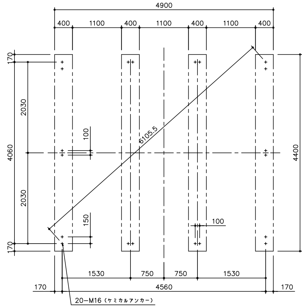
基礎伏図
