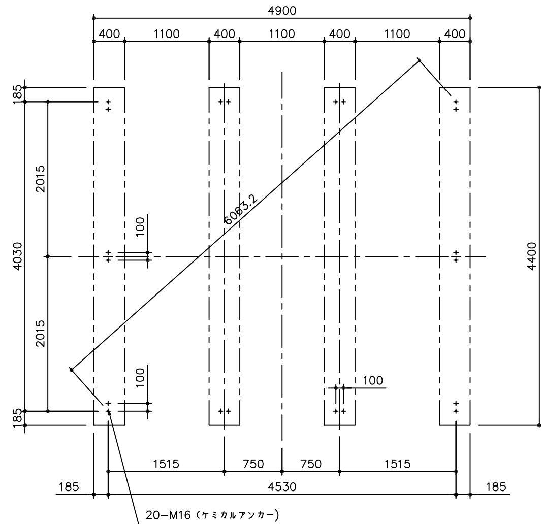
基礎伏図
