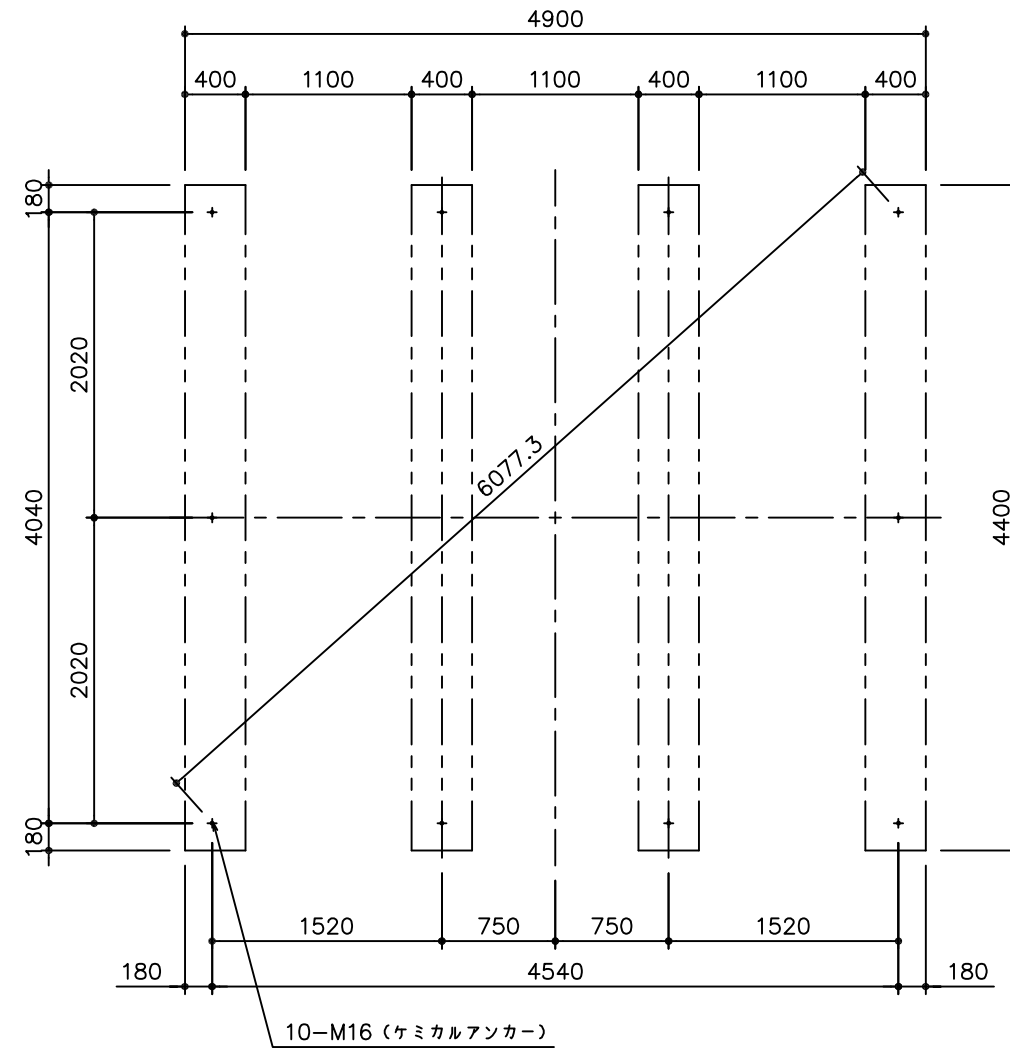
基礎伏図
