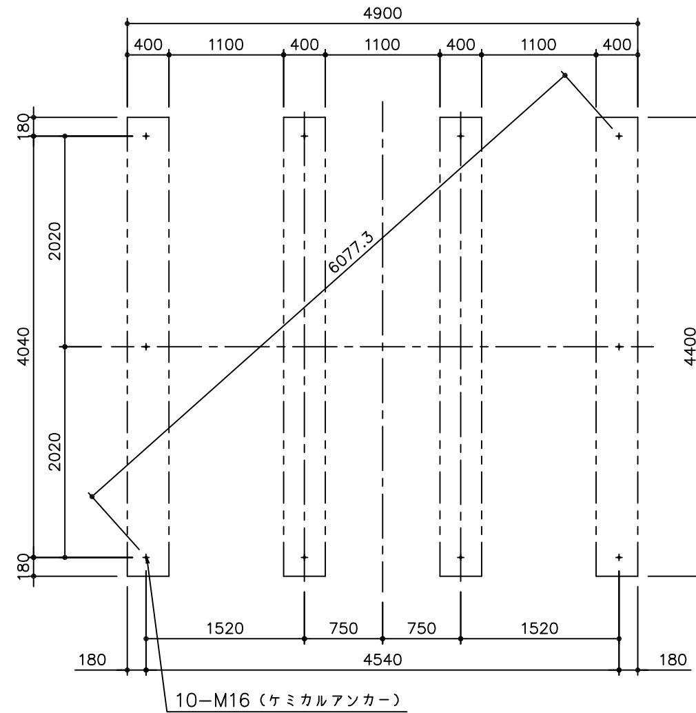
基礎伏図
