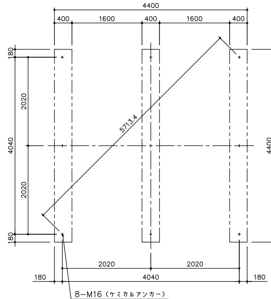
基礎伏図
