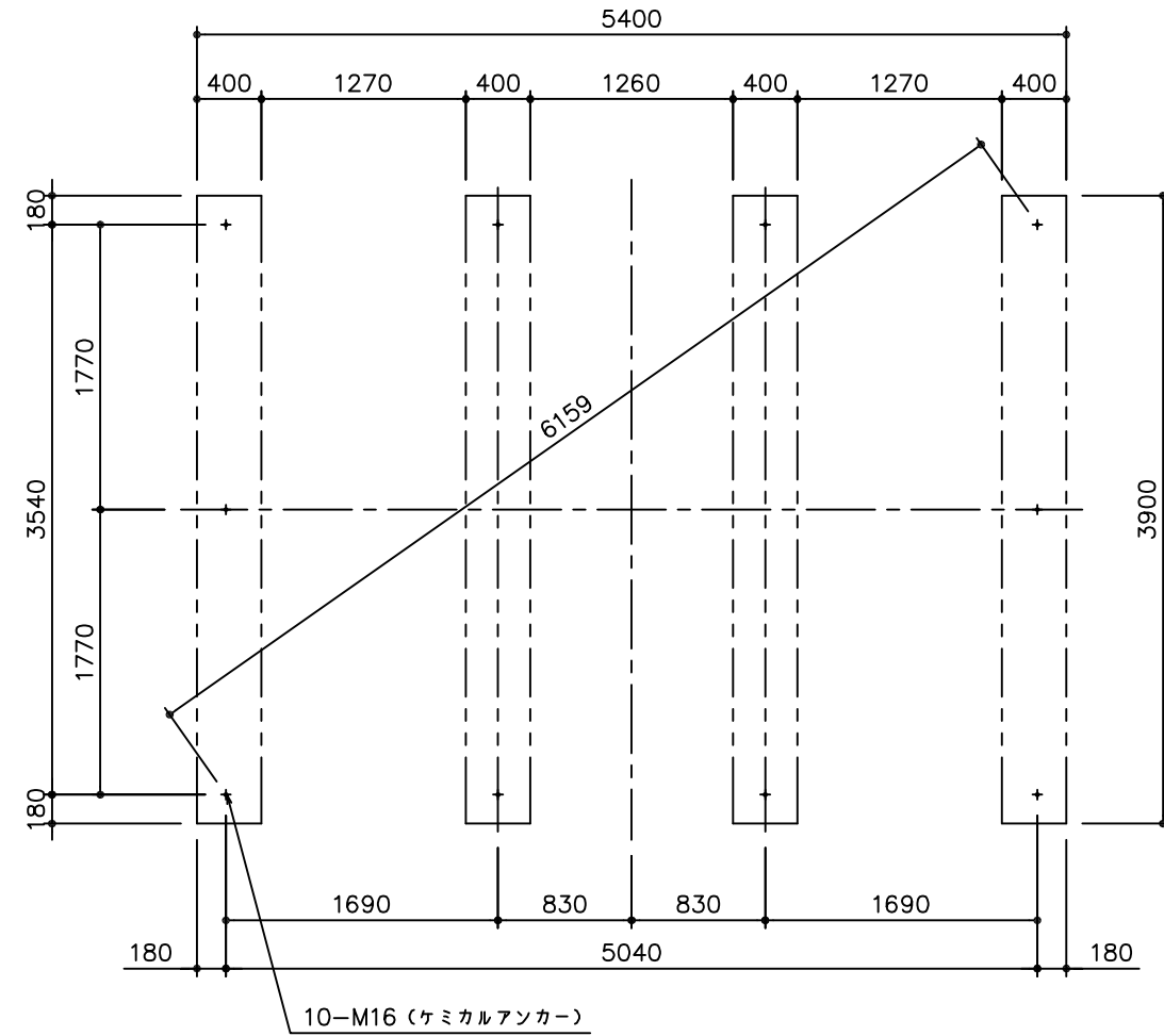
基礎伏図
