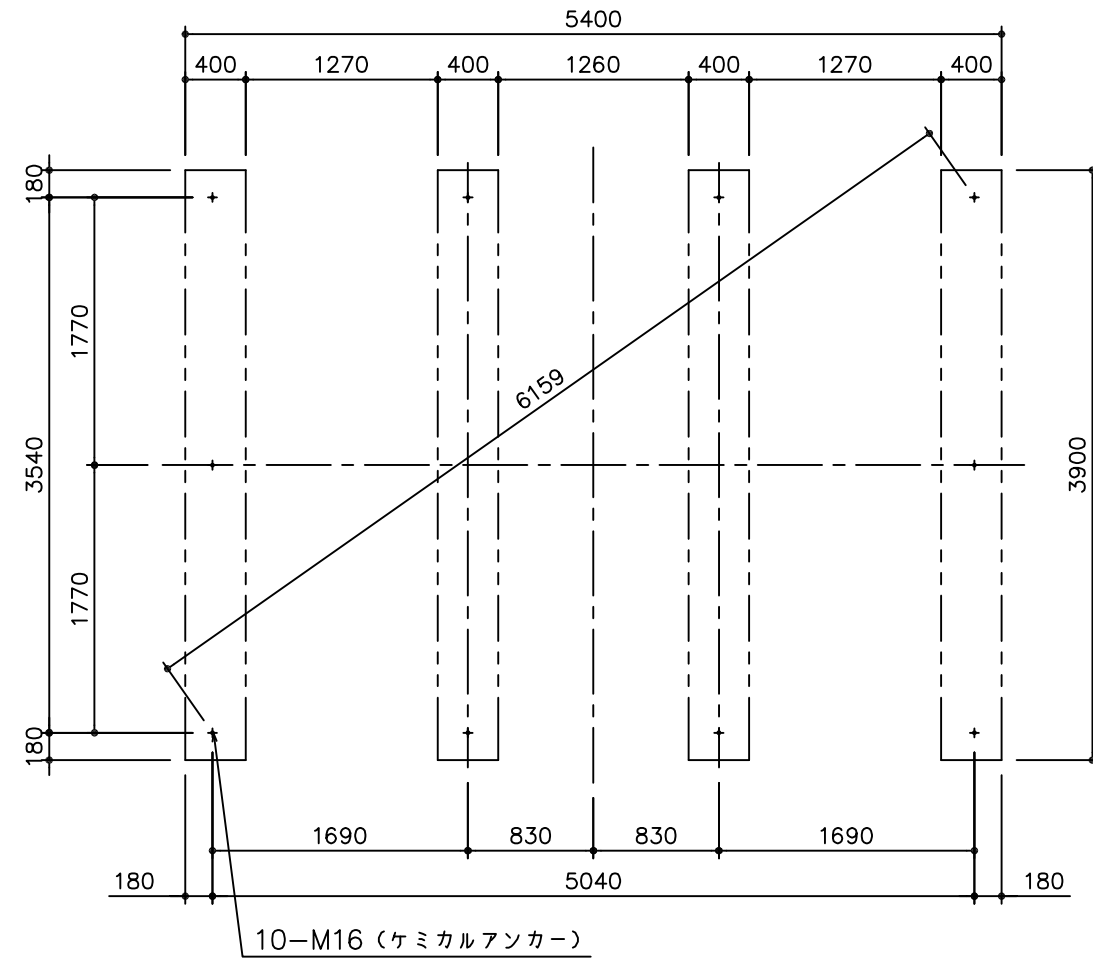
基礎伏図
