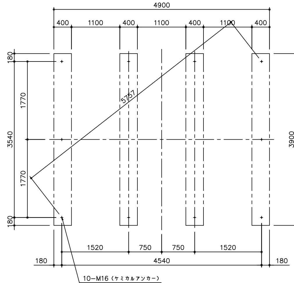
基礎伏図
