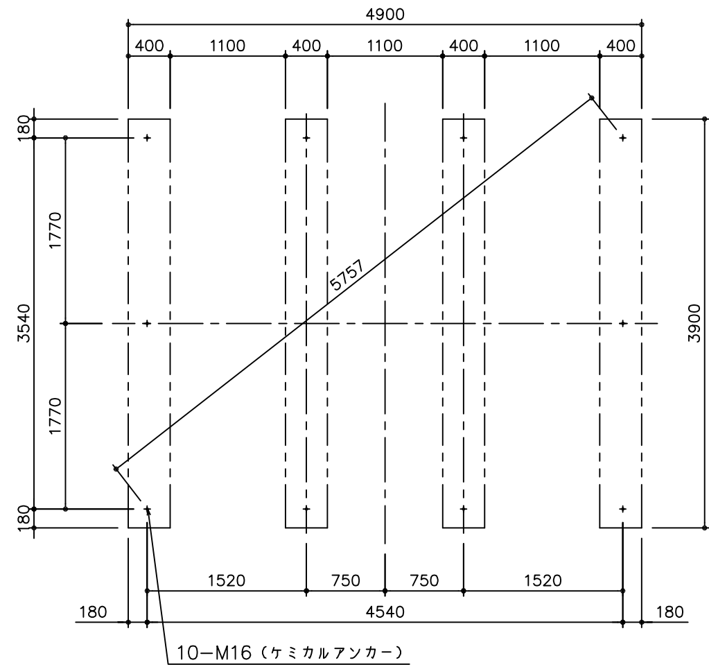
基礎伏図
