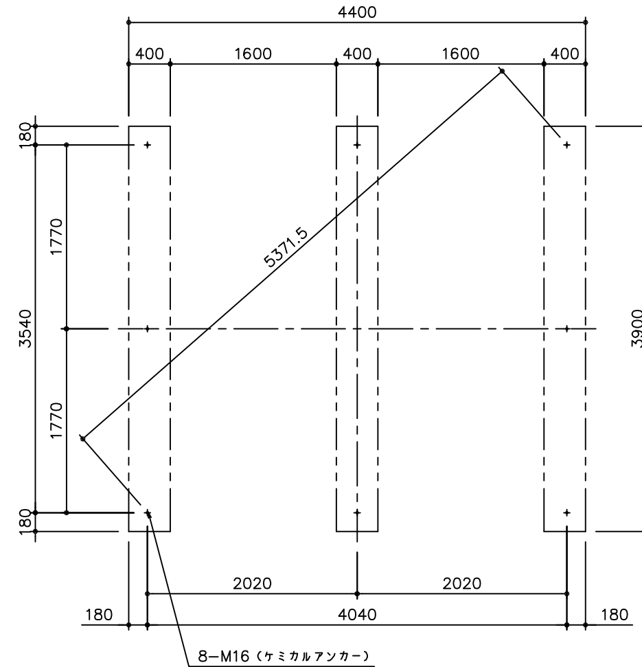
基礎伏図
