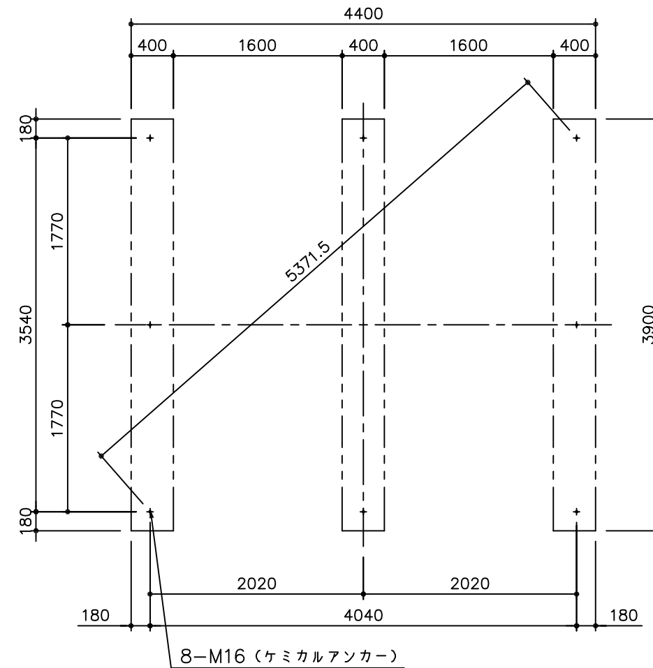
基礎伏図
