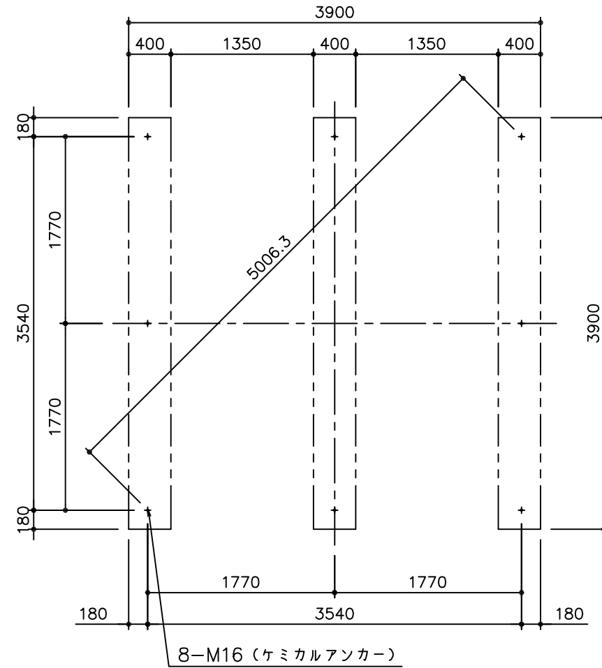
基礎伏図
