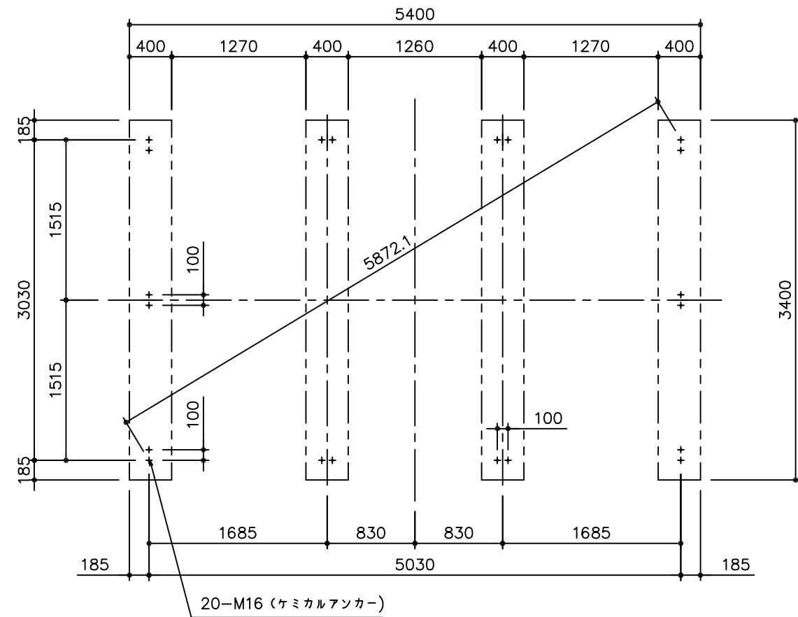
基礎伏図
