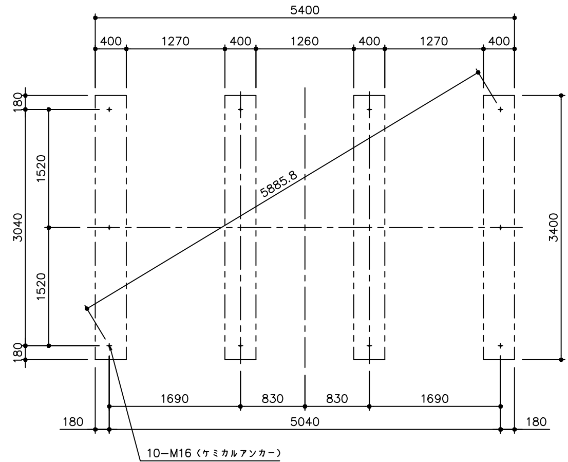
基礎伏図
