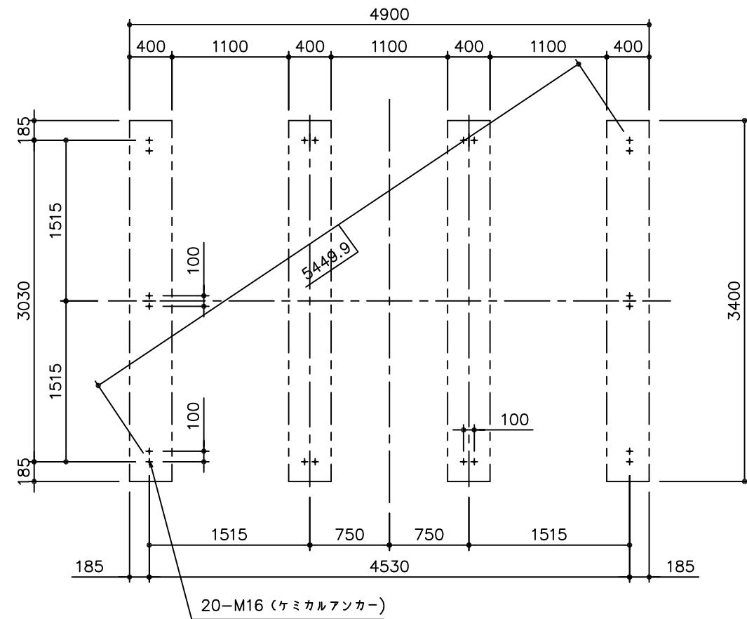
基礎伏図
