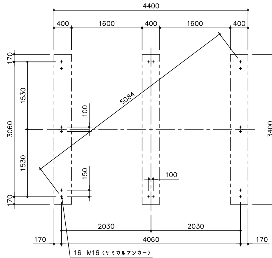
基礎伏図
