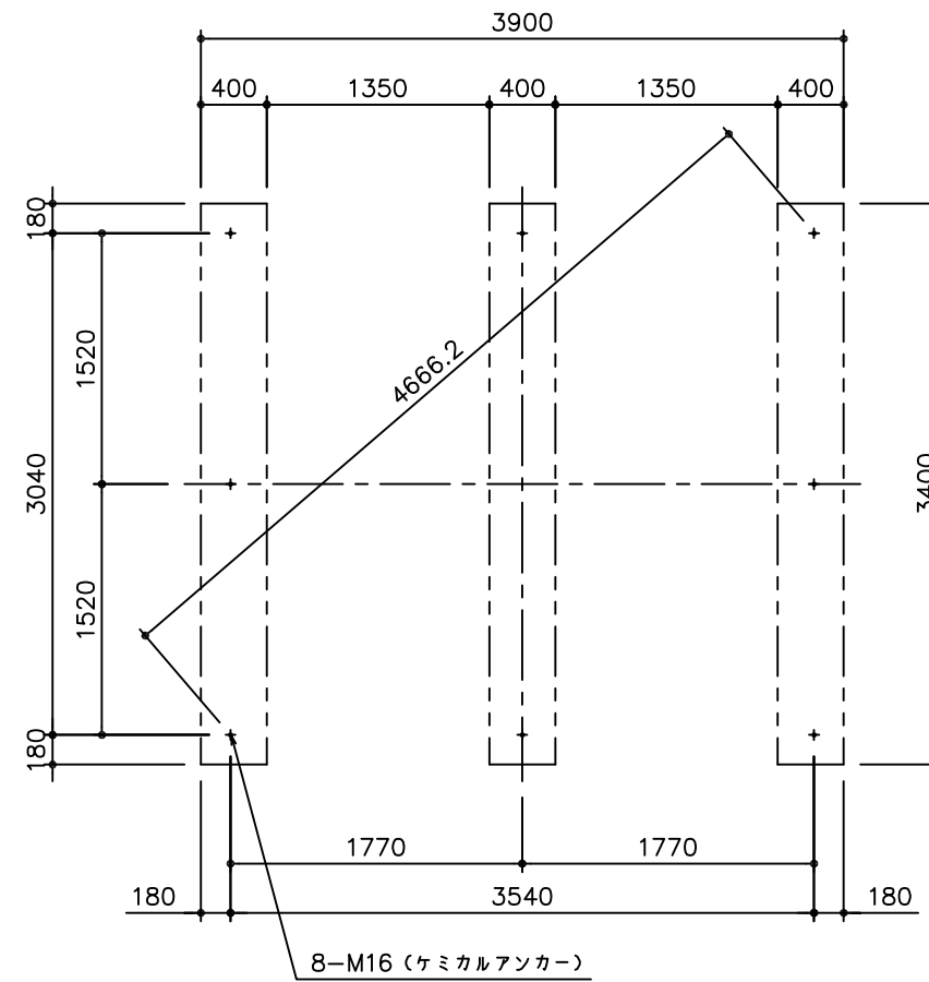
基礎伏図
