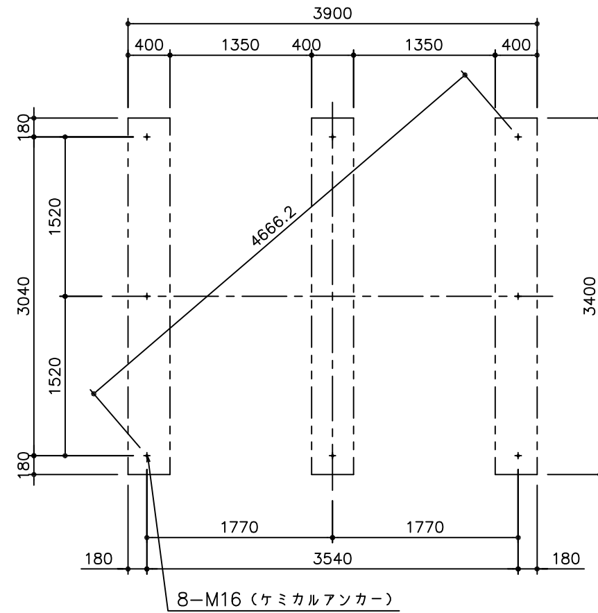
基礎伏図
