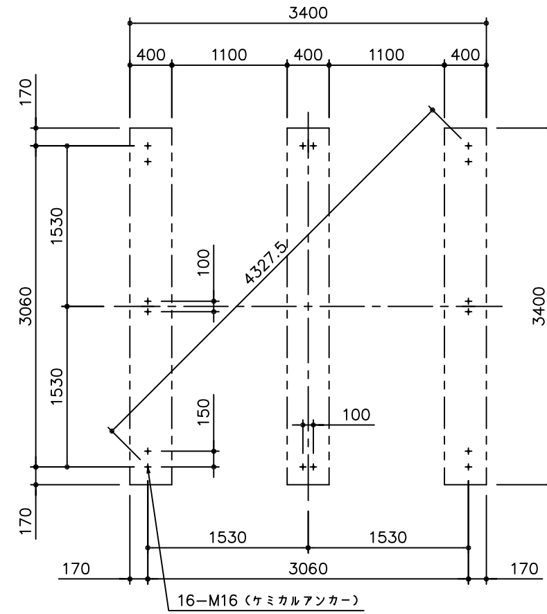
基礎伏図
