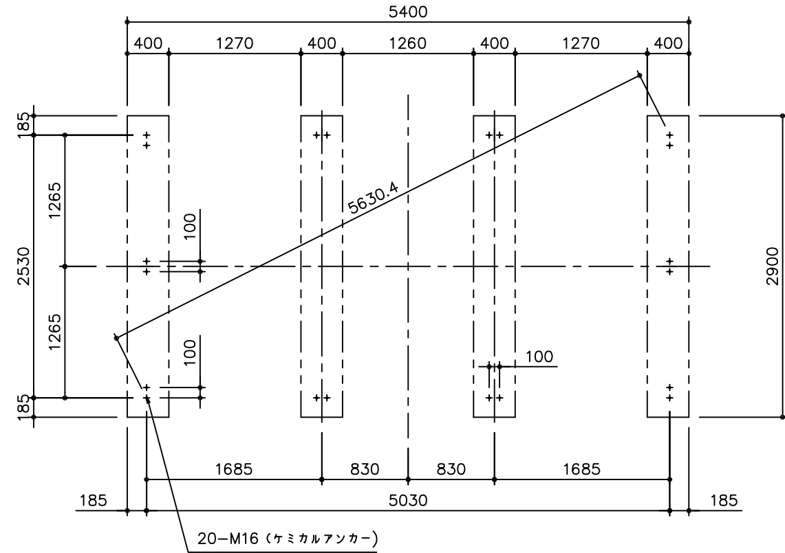
基礎伏図
