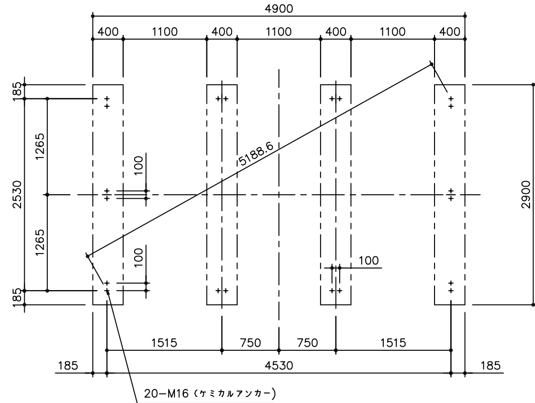
基礎伏図
