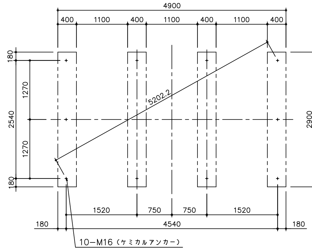
基礎伏図
