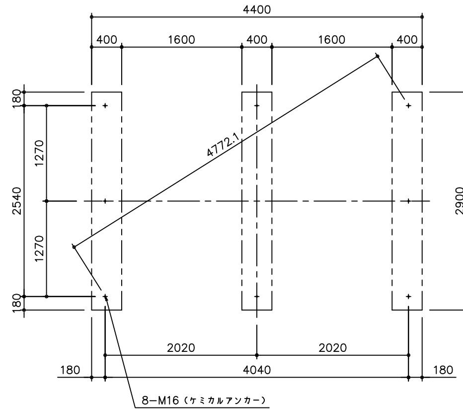
基礎伏図
