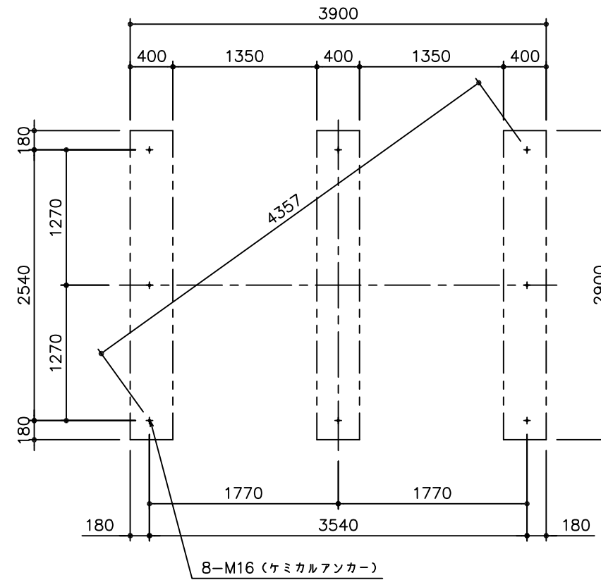
基礎伏図
