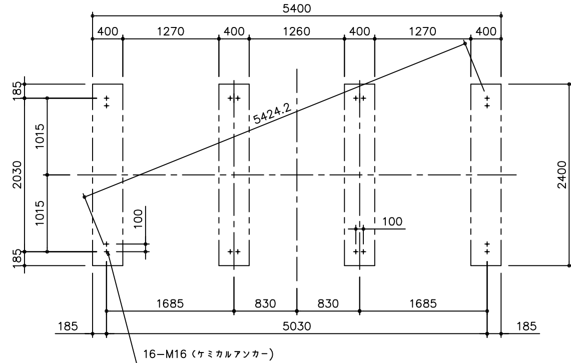
基礎伏図
