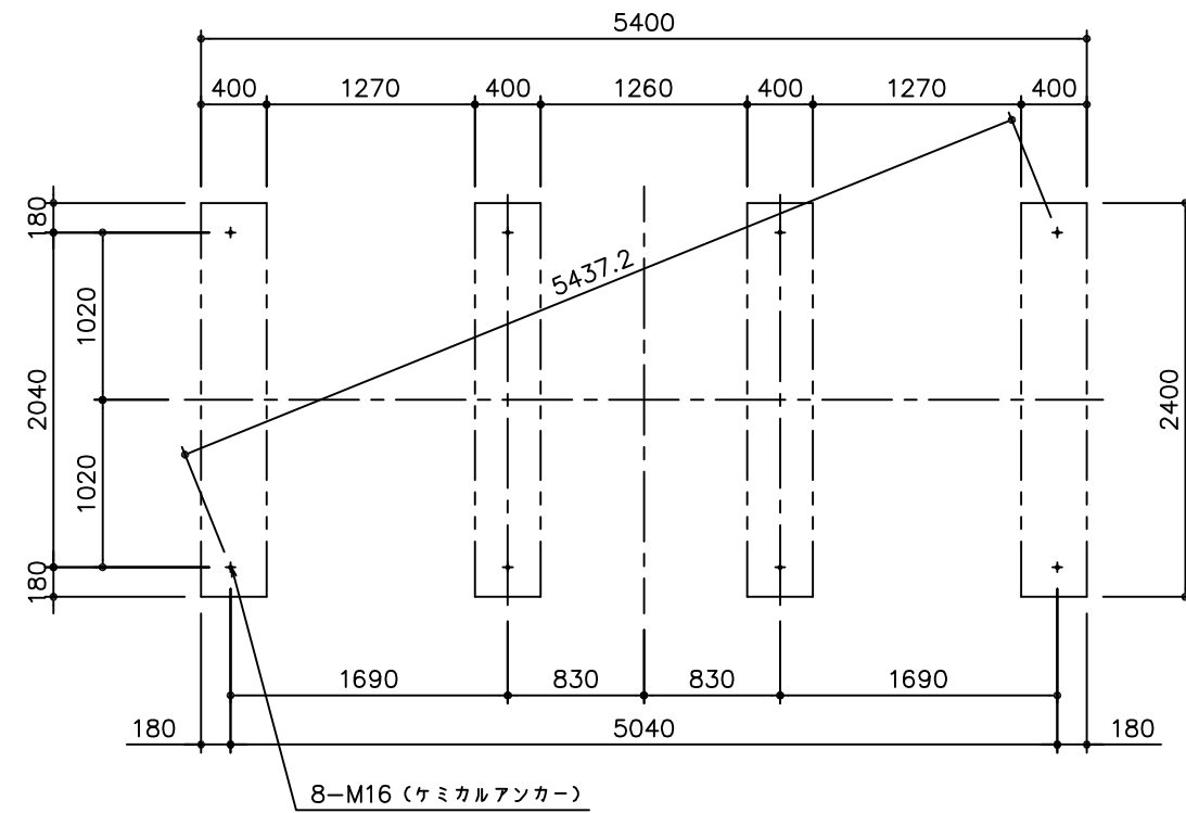
基礎伏図
