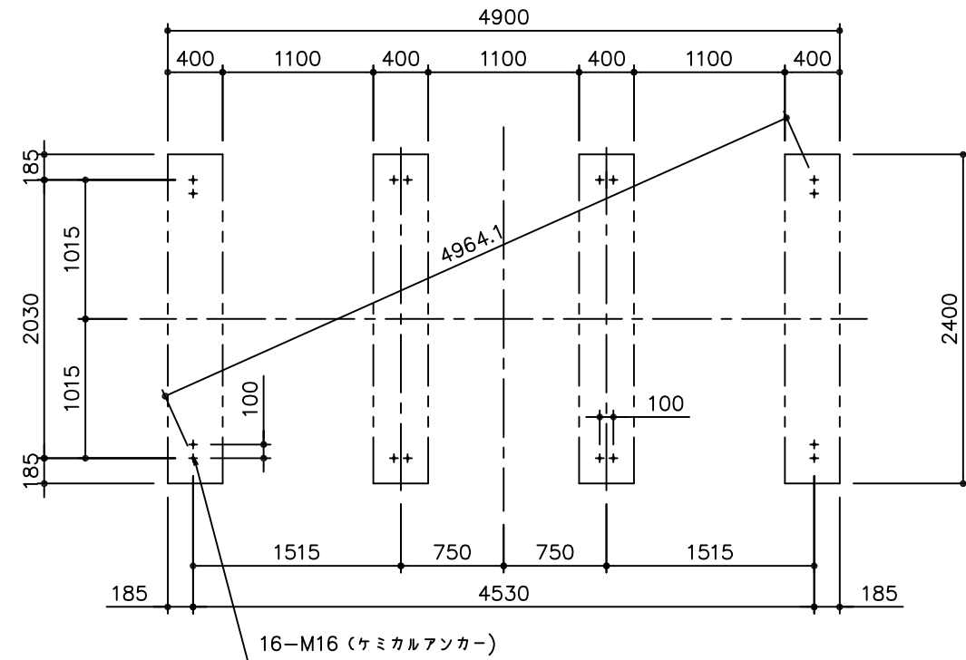
基礎伏図
