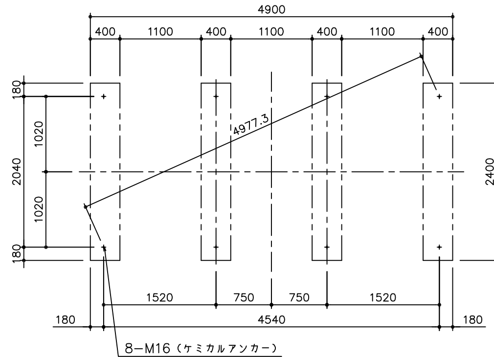
基礎伏図
