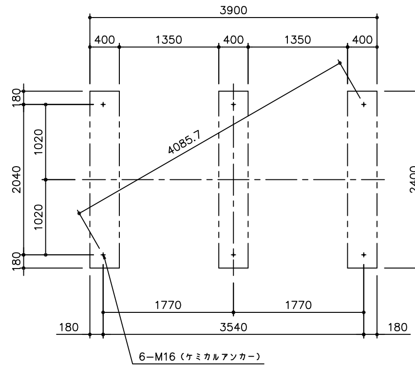
基礎伏図
