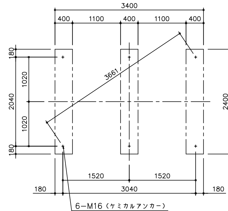
基礎伏図
