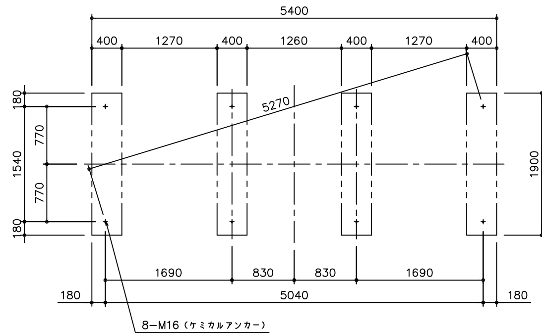
基礎伏図
