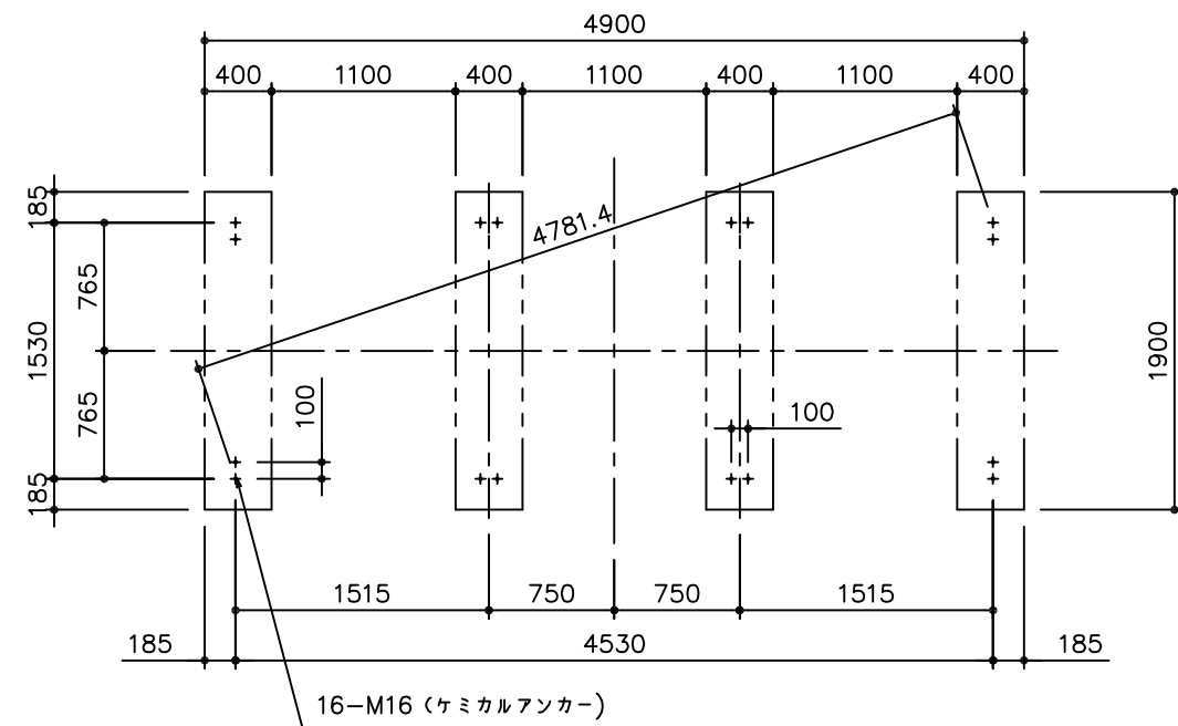
基礎伏図
