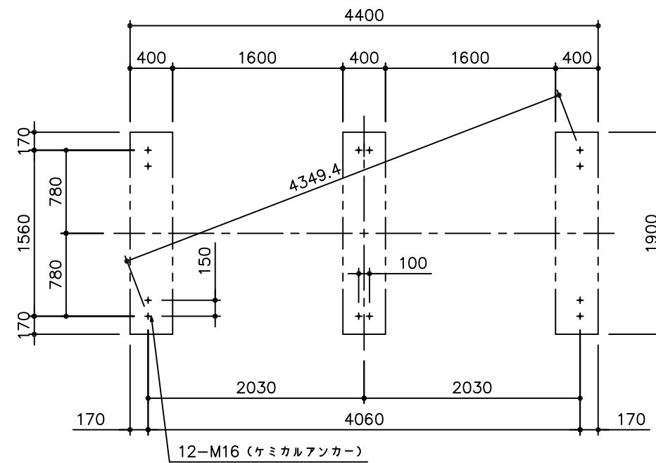
基礎伏図
