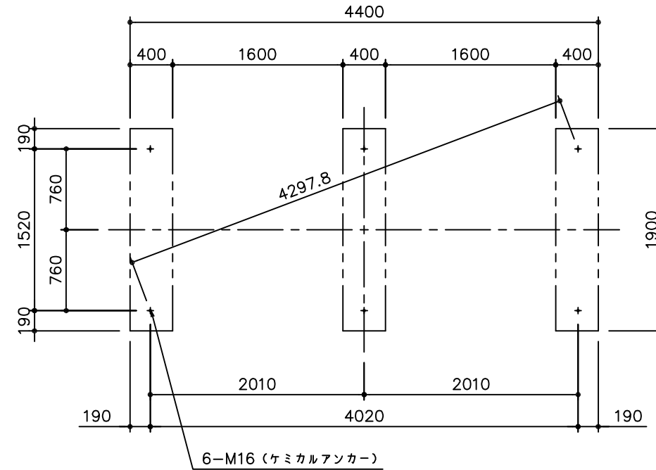
基礎伏図
