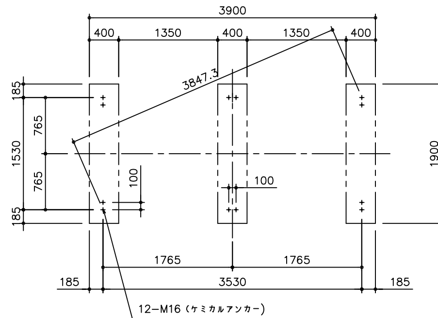
基礎伏図
