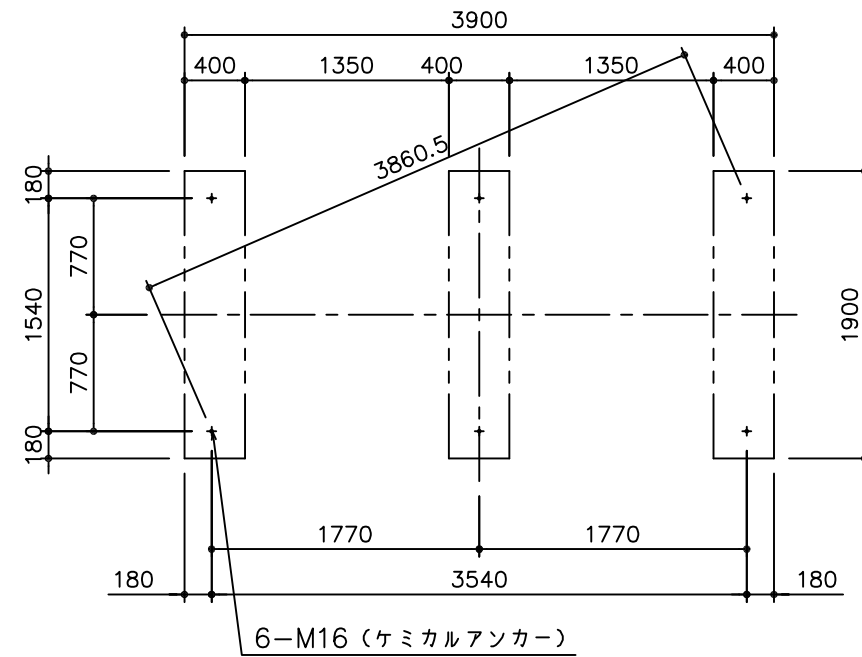
基礎伏図
