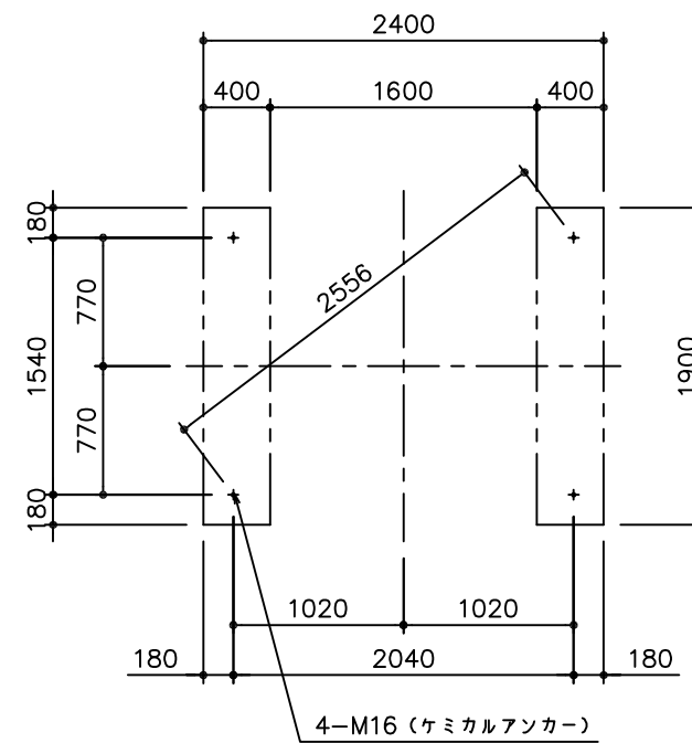
基礎伏図
