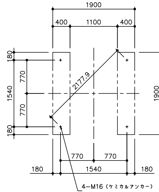
基礎伏図
